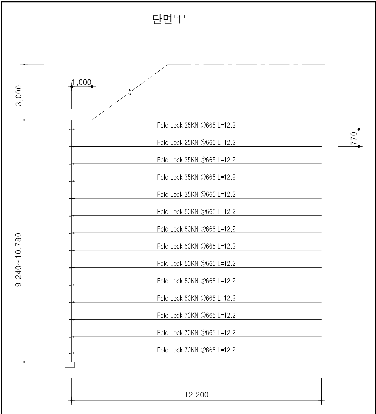
【그림 78.10】 검토단면도
