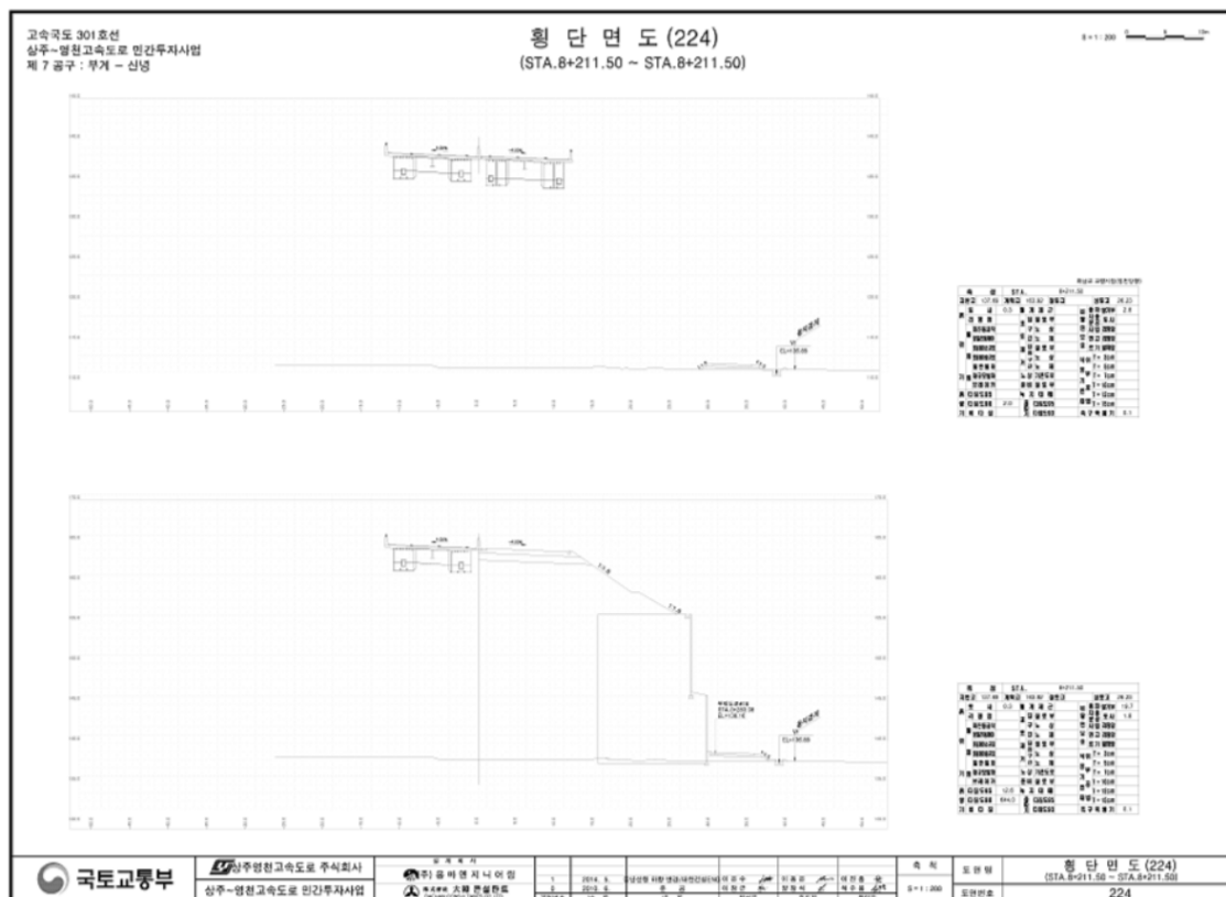
【그림 78.5】 단면도
